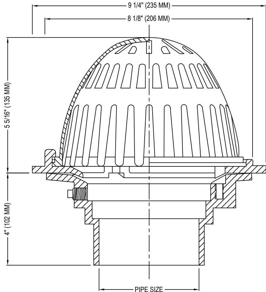
ELEVATION
